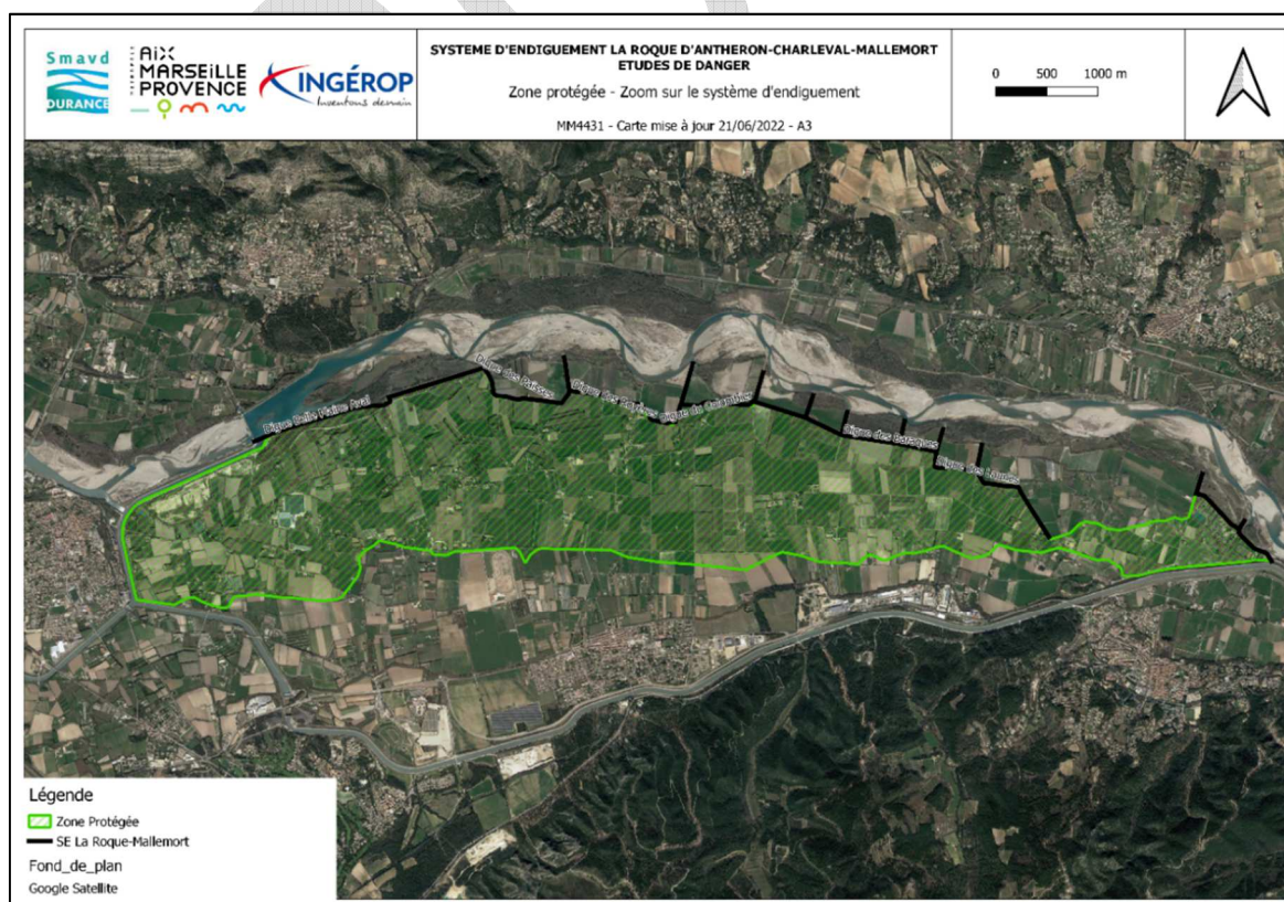
Zone protégée – Zoom à échelle du système d'endiguement
